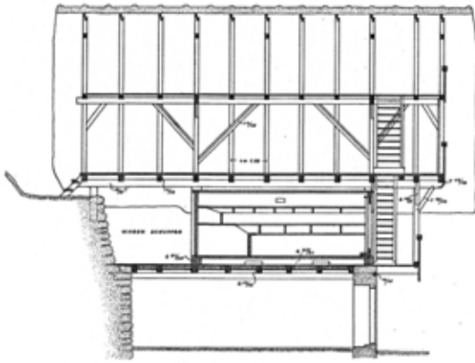
19 Abb. 19: Venturehof, Oberwolfach, Längsschnitt (Zeichnung: Regierungspräsidium Freiburg, Referat 25 – Denkmalpflege, Archivbestand Film-Nr./Bild-Nr. 107/132)
