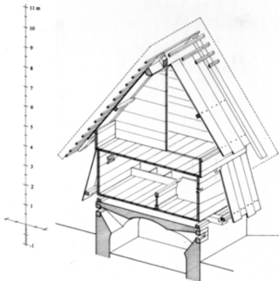
15 Christhofspeicher, St. Georgen-Sommerau. Axonometrische Teilrekonstruktion (Zeichnung: Stefan Blum, 2003, ohne Maßstab)
