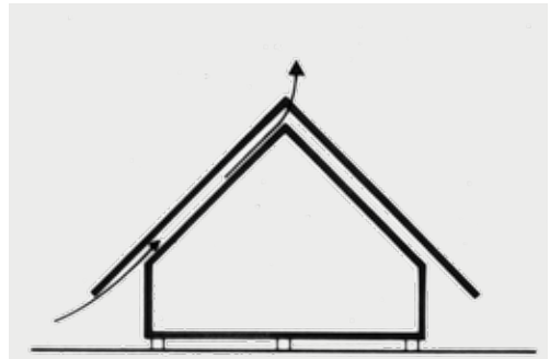
9 Konstruktive Charakteristika, Lagerklima. Doppeldach (Zeichnung: Stefan Blum, 2003)
