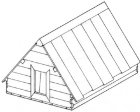
5 Kornkasten mit 5-eckigem Quer-schnitt
