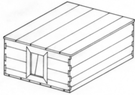
6 Kornkasten mit 4-eckigem Querschnitt (Zeichnungen: Stefan Blum, 2003)
