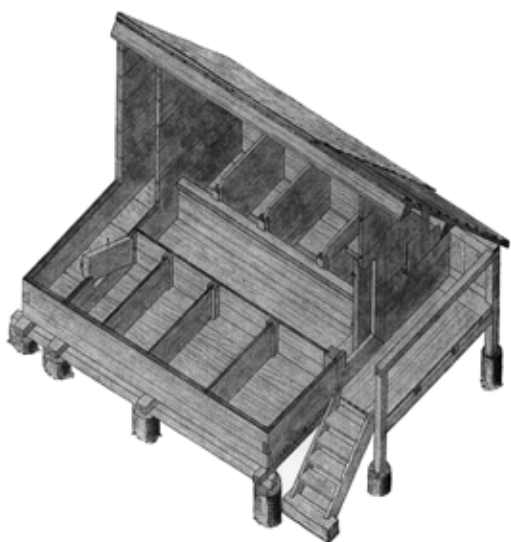
14 G'halt eines im Querschnitt 5-eckigen Kornkastens (Zeichnung: Hermann Schilli: Das Schwarzwaldhaus , Stuttgart 1953, S. 216)
